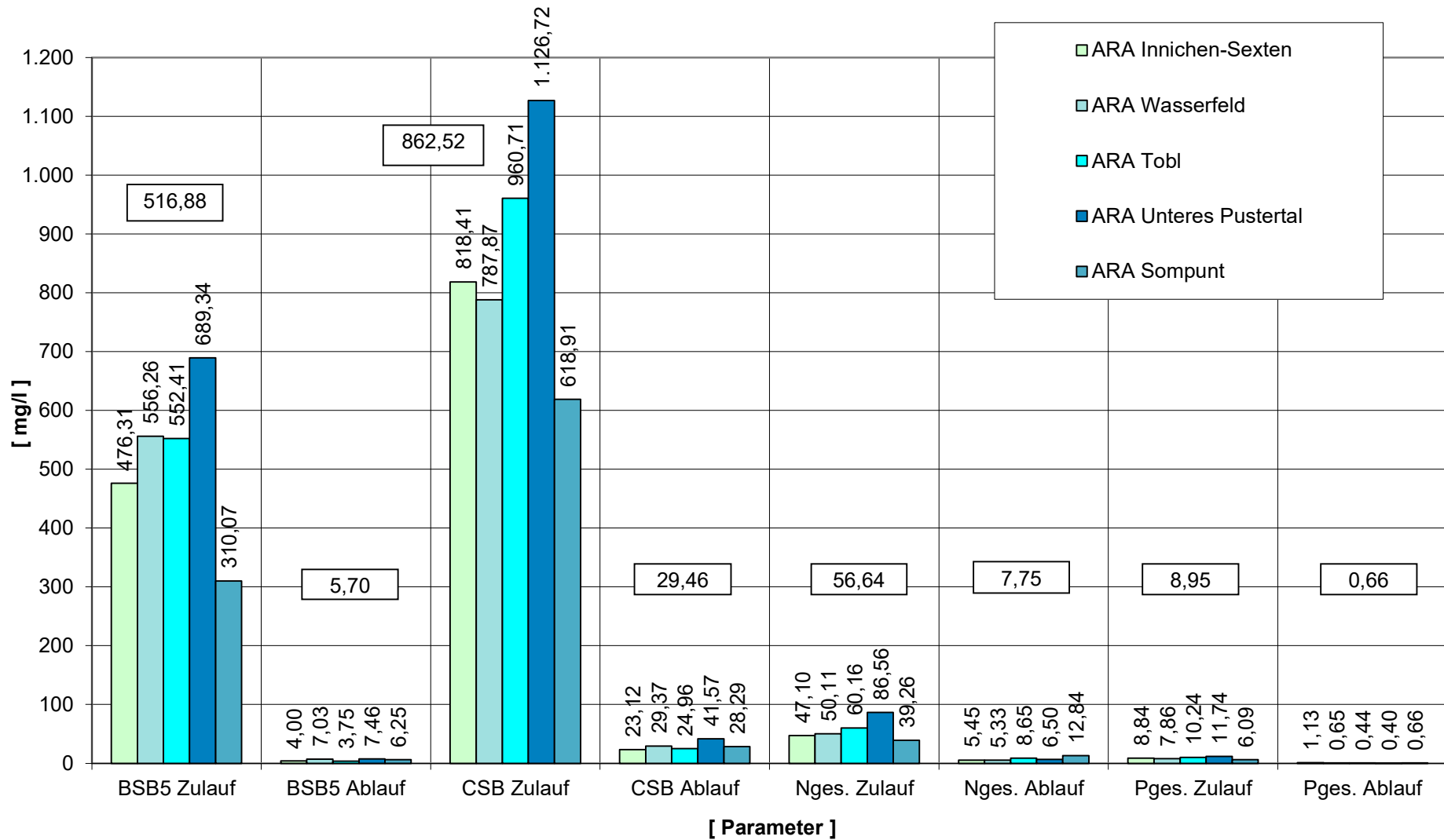
Vergleich der Zu- und Ablaufkonzentrationen der gesetzlichen Parameter; Jahr 2022
