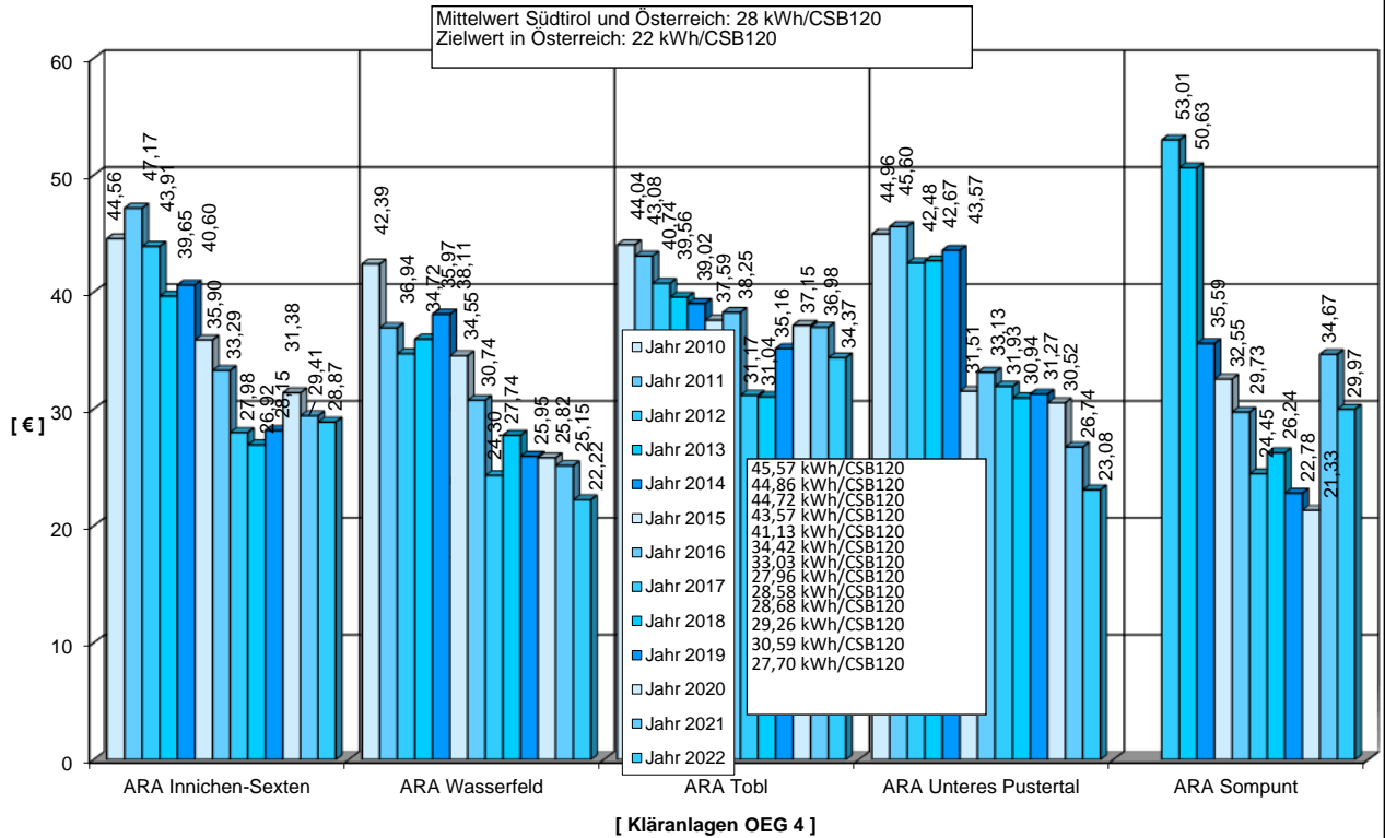
Vergleich des spezifischen Strombedarfes pro EW CSB120 : Jahre 2010-2022
